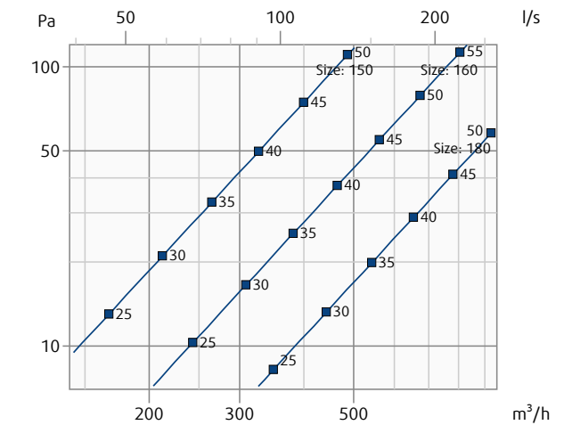
FDR-3G-...-H0
