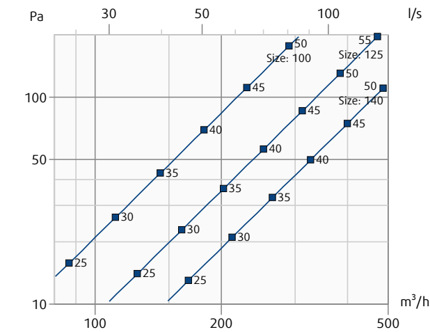
FDR-3G-...-H0
